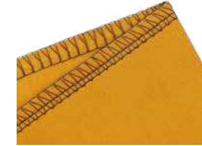
3-Faden-Overlocknaht Versäuberung offener Stoffkanten
